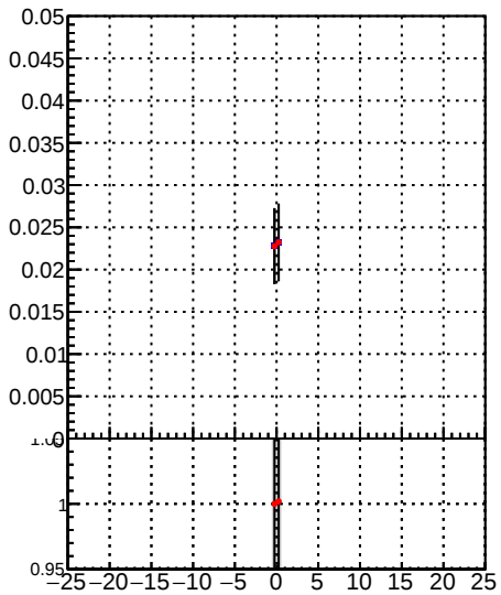
Fake rate vs d —•— DQM TT mkFit-DQM_orig —•— DQM TT mkFit-DQM_mod
