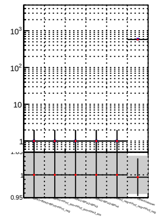
N of reco track vs. \chi^2 —•— DQM TT mkFit-DQM_orig —•— DQM TT mkFit-DQM_mod
