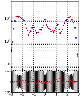
—●— DQM TT mkFit-DQM_orig —●— DQM TT mkFit-DQM_mod
