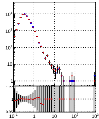
—●— DQM TT mkFit-DQM_orig —●— DQM TT mkFit-DQM_mod
