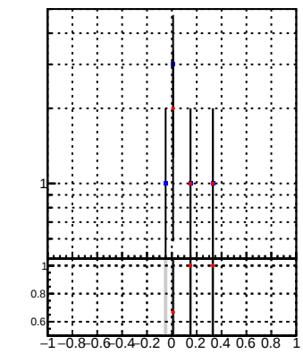
xy(PV)
