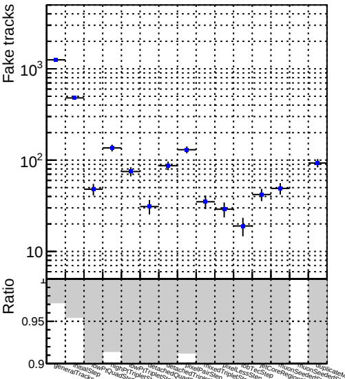
Number DQM_TT__original 1 0.000000 2 0.000000 3 0.000000 4 0.000000 5 0.000000 6 0.000000 7 0.000000 8 0.000000 9 0.000000 10 0.000000 11 0.000000 12 0.000000 13 0.000000 14 0.000000 15 0.000000 16 0.000000 17 0.000000 18 0.000000 19 0.000000 20 0.000000 21 0.000000 22 0.000000 23 0.000000 24 0.000000 25 0.000000 26 0.000000 27 0.000000 28 0.000000 29 0.000000 30 0.000000 31 0.000000 32 0.000000 33 0.000000 34 0.000000 35 0.000000 36 0.000000 37 0.000000 38 0.000000 39 0.000000 40 0.000000 41 0.000000 42 0.000000 43 0.000000 44 0.000000 45 0.000000 46 0.000000 47 0.000000 48 0.000000 49 0.000000 50 0.000000 51 0.000000 52 0.000000 53 0.000000 54 0.000000 55 0.000000 56 0.000000 57 0.000000 58 0.000000 59 0.000000 60 0.000000 61 0.000000 62 0.000000 63 0.000000 64 0.000000 65 0.000000 66 0.000000 67 0.000000 68 0.000000 69 0.000000 70 0.000000 71 0.000000 72 0.000000 73 0.000000 74 0.000000 75 0.000000 76 0.000000 77 0.000000 78 0.000000 79 0.000000 80 0.000000 81 0.000000 82 0.000000 83 0.000000 84 0.000000 85 0.000000 86 0.000000 87 0.000000 88 0.000000 89 0.000000 90 0.000000 91 0.000000 92 0.000000 93 0.000000 94 0.000000 95 0.000000 96 0.000000 97 0.000000 98 0.000000 99 0.000000 100 0.000000 101 0.000000 102 0.000000 103 0.000000 104 0.000000 105 0.000000 106 0.000000 107 0.000000 108 0.000000 109 0.000000 110 0.000000 111 0.000000 112 0.000000 113 0.000000 114 0.000000 115 0.000000 116 0.000000 117 0.000000 118 0.000000 119 0.000000 120 0.000000 121 0.000000 122 0.000000 123 0.000000 124 0.000000 125 0.000000 126 0.000000 127 0.000000 128 0.000000 129 0.000000 130 0.000000 131 0.000000 132 0.000000 133 0.000000 134 0.000000 135 0.000000 136 0.000000 137 0.000000 138 0.000000 139 0.000000</
