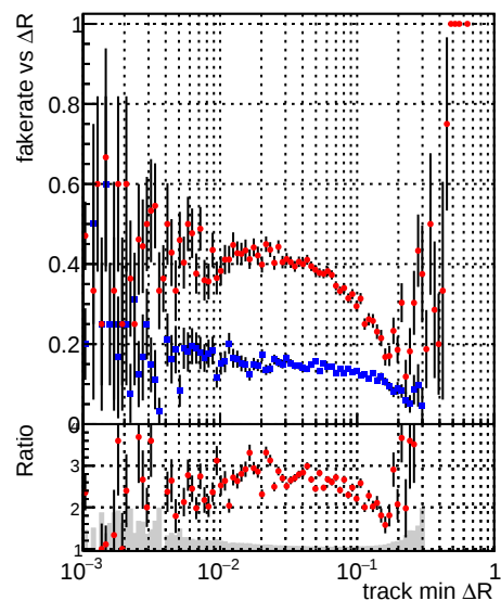
■ DQM_TTbarTEST ◆ DQM_mkFitTTbarTEST
