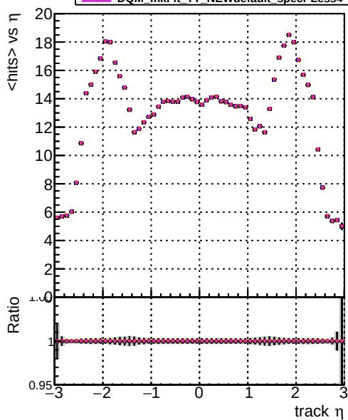
Legend: DQM mkFit TT NEWdefault specPless1, DQM mkFit TT NEWdefault specPless2, DQM mkFit TT NEWdefault specPless3, DQM mkFit TT NEWdefault specPless4 mean hits
