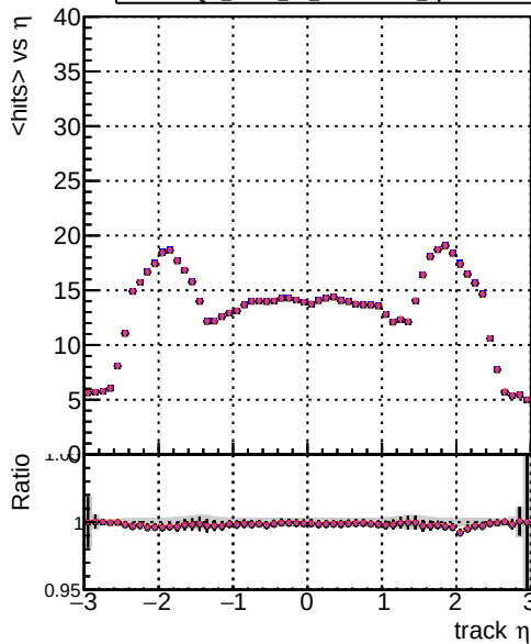
mean hits DQM mkFit TT NEWdefault specPless1 DQM mkFit TT NEWdefault specPless2 DQM mkFit TT NEWdefault specPless3 DQM mkFit TT NEWdefault specPless4
