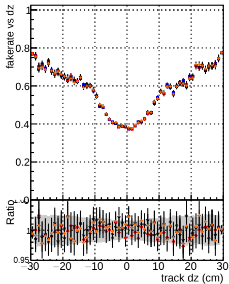
—•— DQM mkFit TToriginal —•— DQM mkFit TTnewMS-genMatch-CUT2 —•— DQM mkFit TTnewMS-genMatch-CUT2
