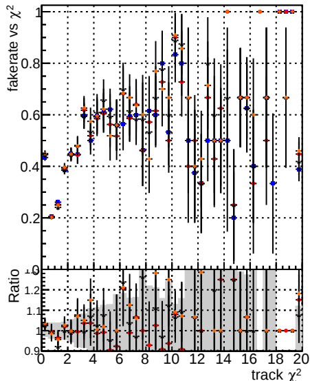
Fake rate vs. \chi^2 for DQM mkFit, DQM mkFit + TopVeto, and DQM mkFit + TopVeto + genMatch-CUT2
