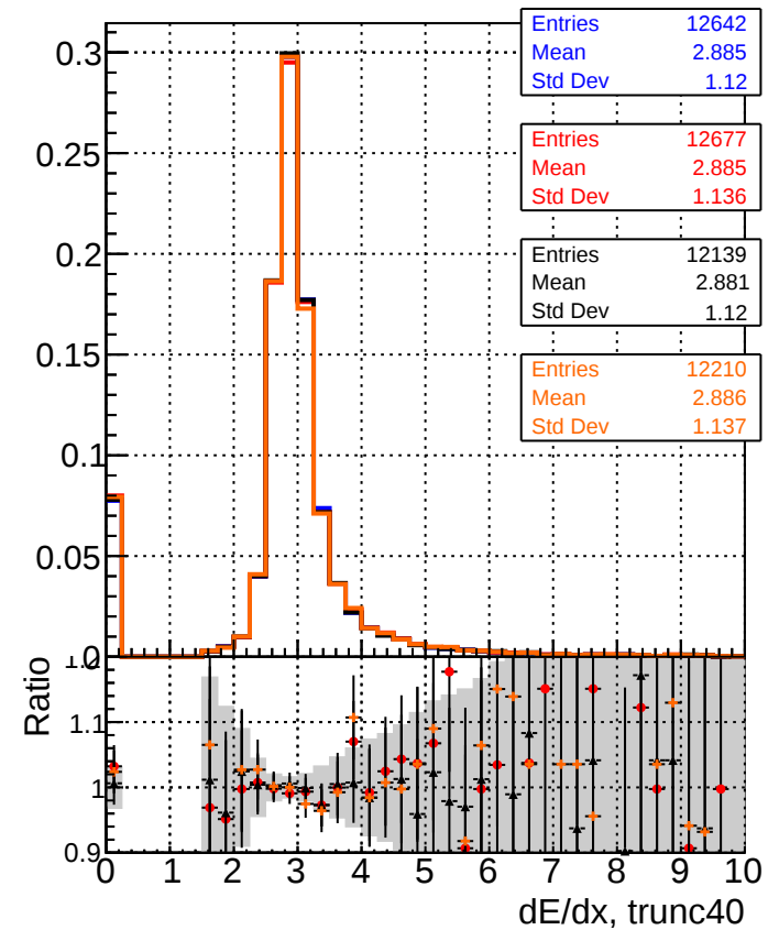
dE/dx estimator 2
