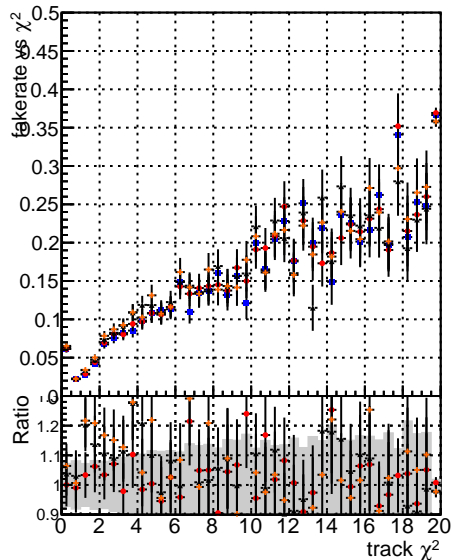
Fake rate vs. █ BGM mkFit T-Original █ BGM mkFit T-NEWMS █ BGM mkFit T-REWMS genMatch-CUT2
