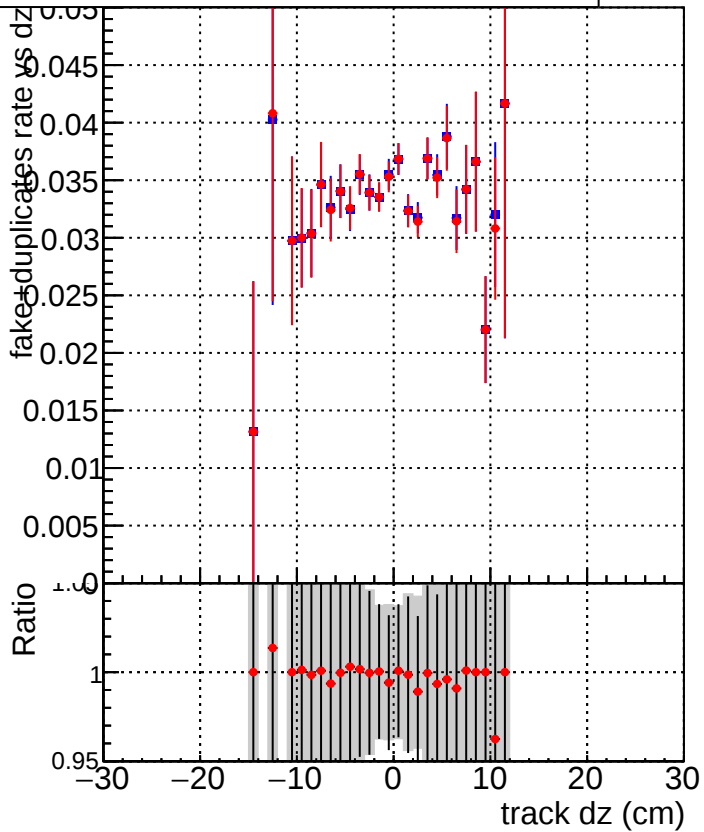
DQM_beforePR DQM_correctCheck
