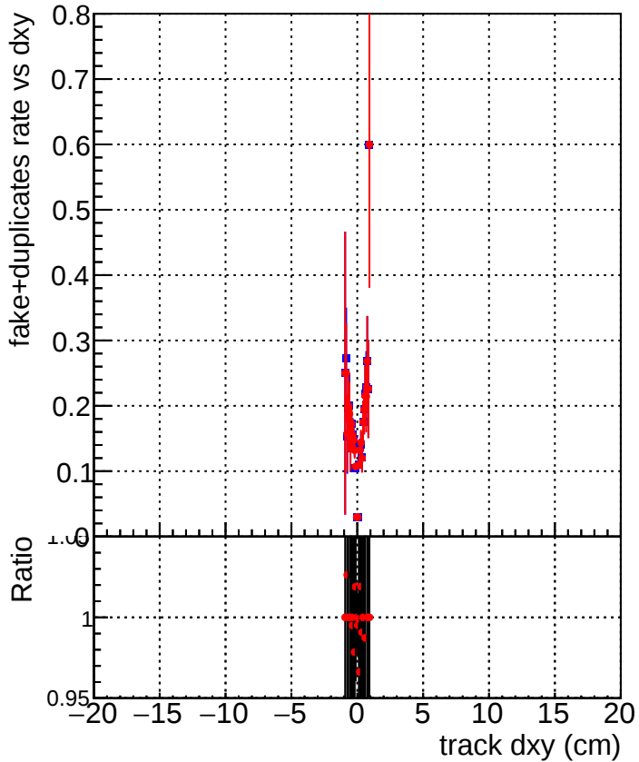
DQM_beforePR DQM_correctCheck
