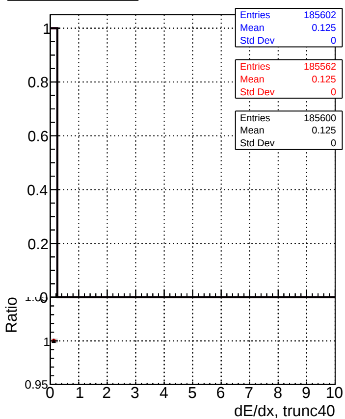
dE/dx estimator 2
