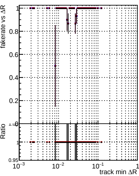
Fake rate vs \Delta R(\text{track, jet}) DQM beforePR DQM afterPR DQM partialCheck
