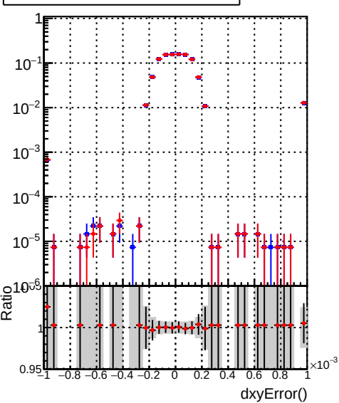
(PackedCandidate::dxyError() - reco::Track::dxyError())/reco::Track
