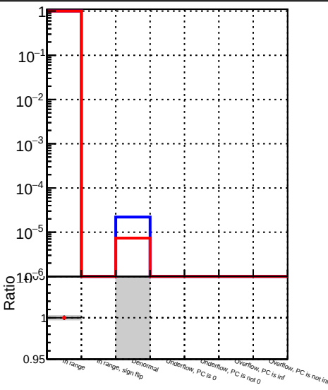
(PackedCandidate::dzError() - reco::Track::dzError())/reco::Track
