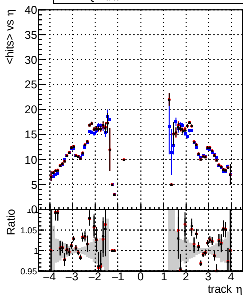
mean hits vs \eta — DQM_noMkFit — DQM_beforePR — DQM_afterPR
