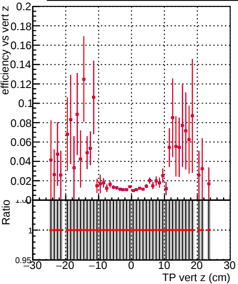
Efficiency vs TP vert z (cm) DQM_beforePR DQM_afterPR
