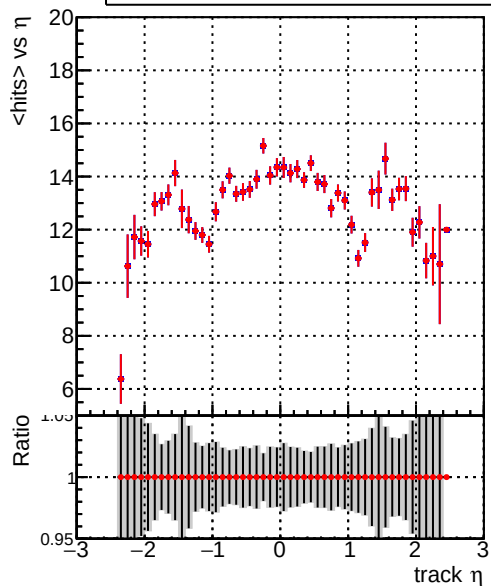
mean hits — DQM_beforePR — DQM_afterPR
