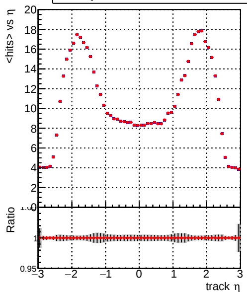
— DQM_beforePR — DQM_afterPR mean hits
