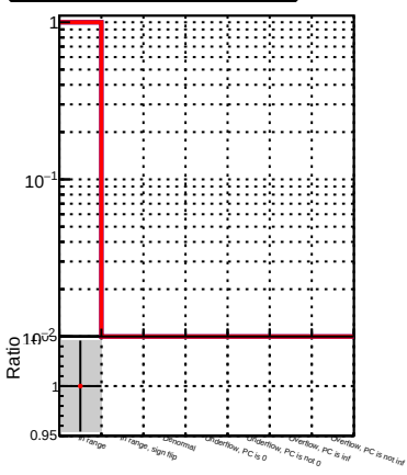
(packedCandidate:bestTrack) - reco:Track(reco:Track in cov(dsz, dsz) status)
