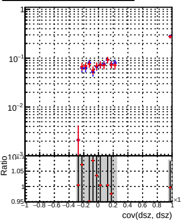
(packedCandidate:bestTrack) - reco:Track(reco:Track in cov(dsz, dsz))
