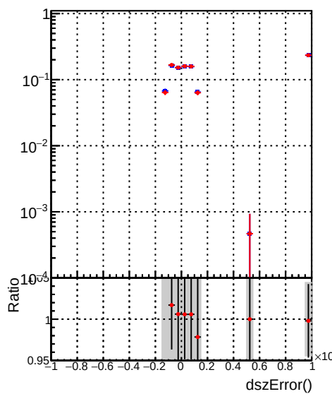
(PackedCandidate::dzError() - reco::Track::dzError())/reco::Track
