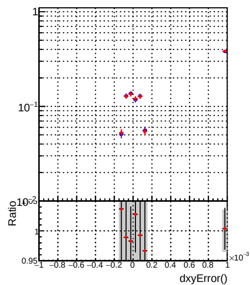
(PackedCandidate::dxyError() - reco::Track::dxyError())/reco::Track
