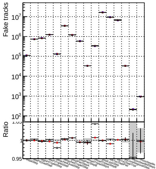
DQM_mkFit_TToriginal DQM_mkFit_TT_JanUpdate-noErr DQM_mkFit_TT_JanUpdate-noErr1H
