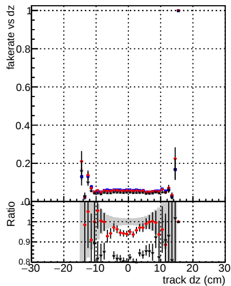
DOM mkFit Toriginal DOM mkFit JanUpdate-noErr DOM mkFit JanUpdate-noErr1H
