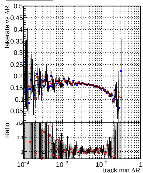
—•— DQM_mkFit_TToriginal —•— DQM_mkFit_TT_JanUpdate-noErr —•— DQM_mkFit_TT_JanUpdate-1H
