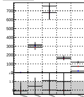
lowPtTripletStep
