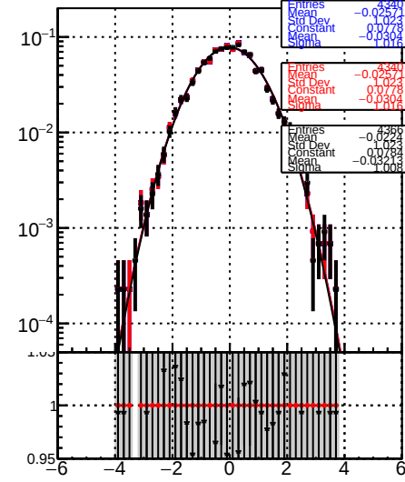
RecoAllAssoc2GenMatched_PulIZ
