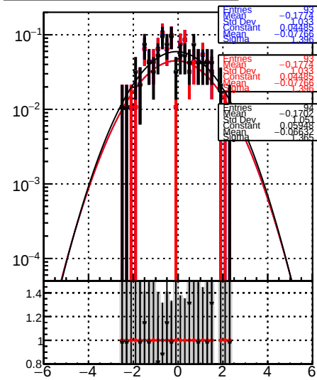
RecoPVAssoc2GenPVMatched_PulIZ
