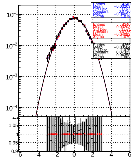
RecoAllAssoc2GenMatched_PulIZ
