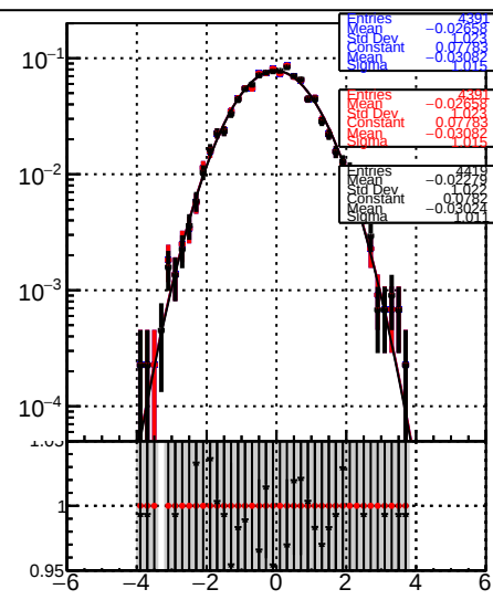
RecoAllAssoc2GenMatched_PulIZ
