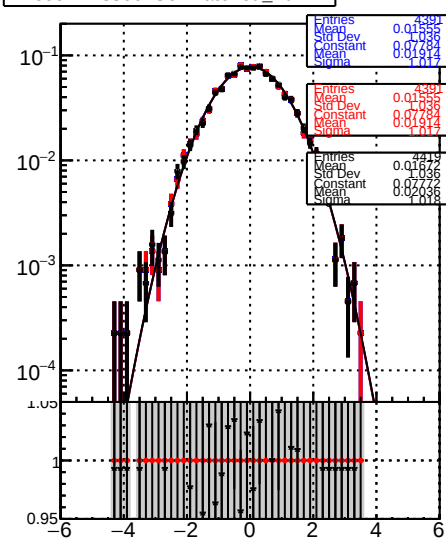
RecoAllAssoc2GenMatched_PulIX
