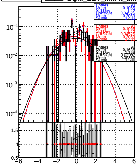
RecoPVAssoc
