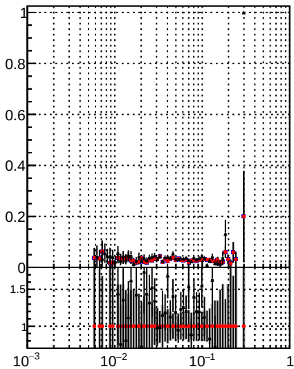
Fake rate vs \sqrt{s} —•— DQM mkFit time —•— DQM mkFit time b1 —•— DQM BDT_mkFit_time
