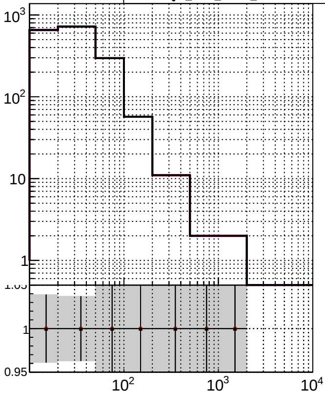
RecoAssoc2GenPVM
