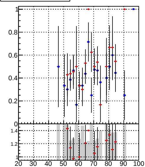
fake+duplicates vs PU
