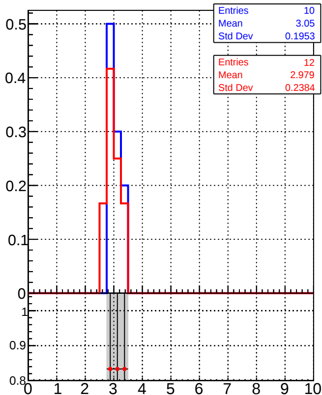
dE/dx estimator 2
