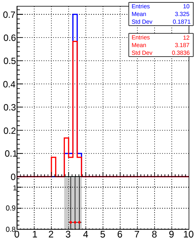
dE/dx estimator 1
