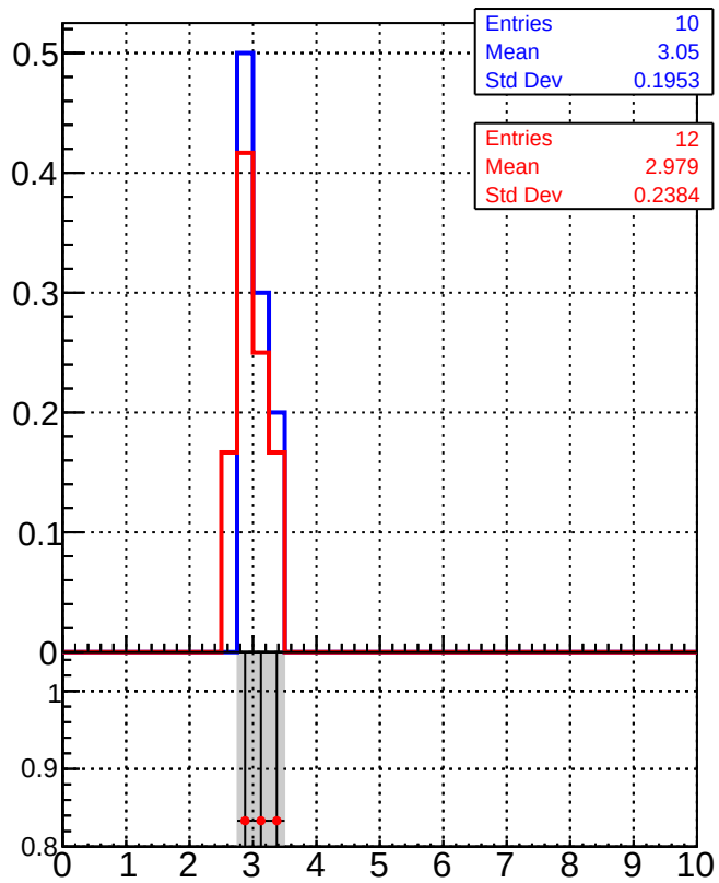
dE/dx estimator 2
