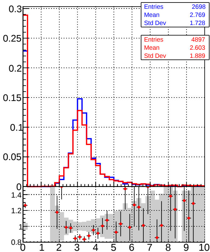
dE/dx estimator 1
