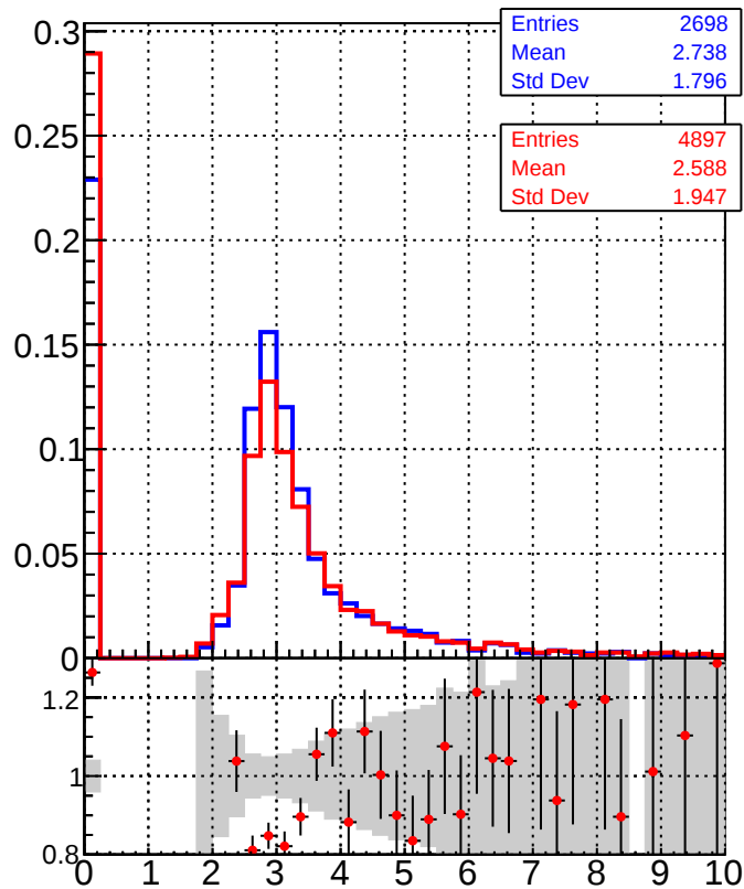
dE/dx estimator 2
