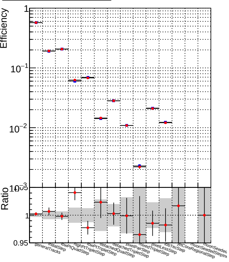
DQM_TT_PR43146 DQM_TT_PR43146_swap
