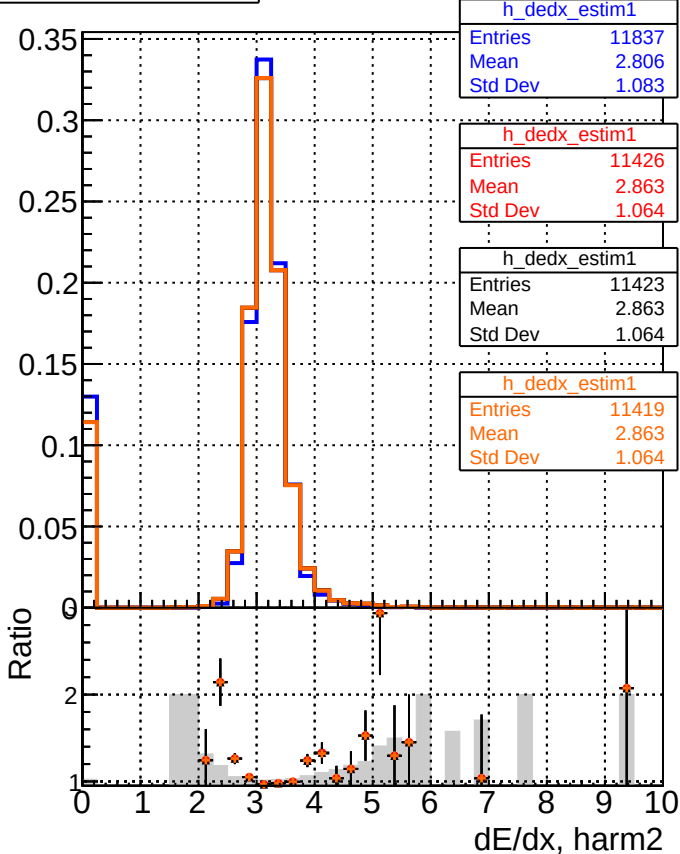
dE/dx estimator 1
