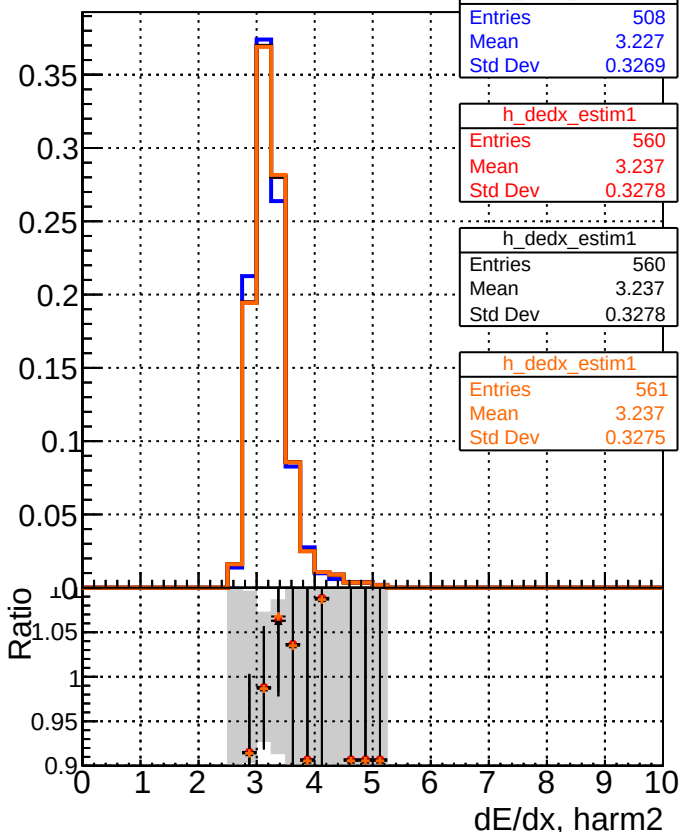
dE/dx estimator 1
