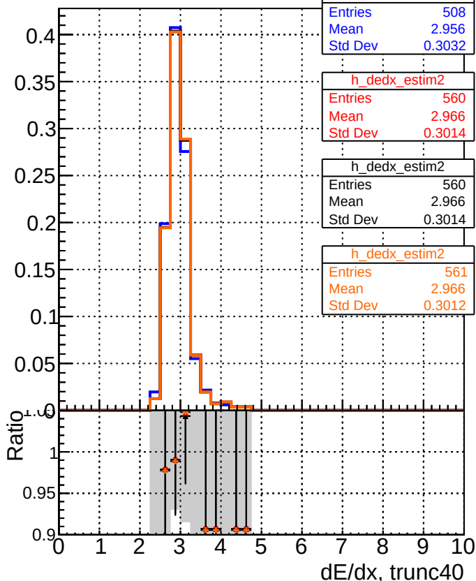
dE/dx estimator 2
