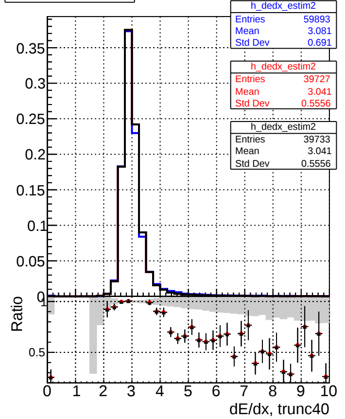
dE/dx estimator 2
