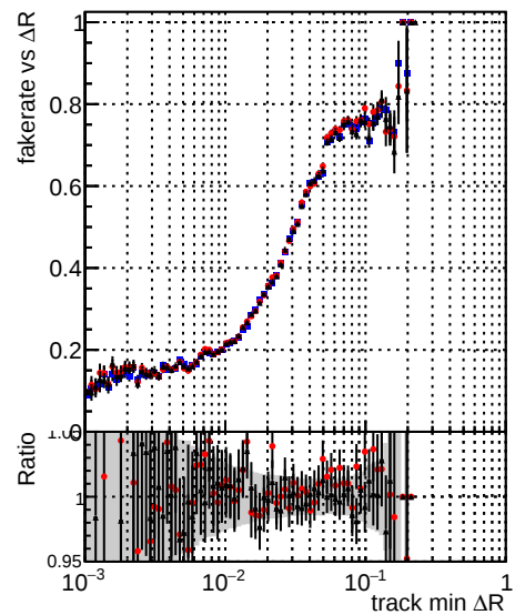
Legend: - \bullet DQM TT original time2 - \bullet DQM TT modified time2 - \bullet DQM TT modified INIT time2
