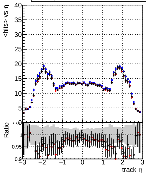
mean hits — DQM_TT_original_time2 — DQM_TT_modified_time2 — DQM_TT_modifiedINIT_time2
