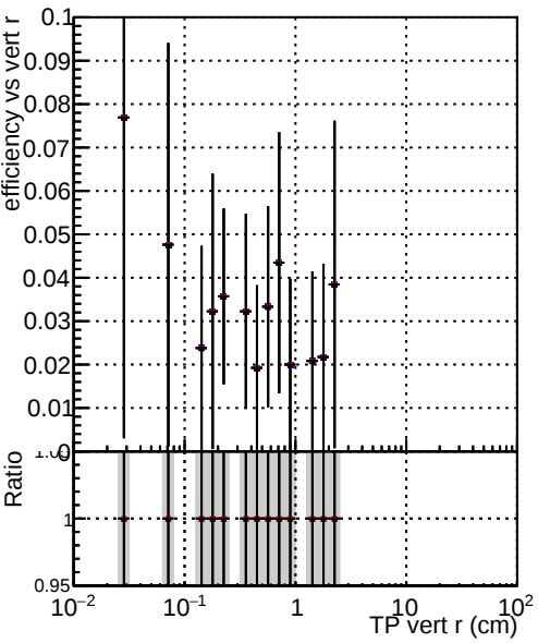
Efficiency vs vertpos DQM_TT_original_time2 DQM_TT_modified_time2 DQM_TT_modifiedINIT_time2
