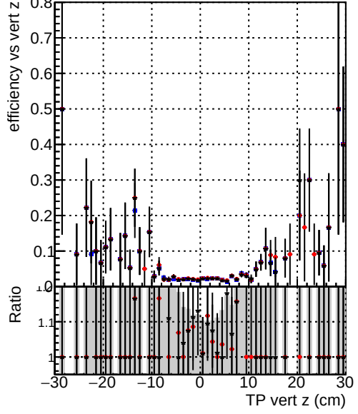
Efficiency vs. TP vert z —●— DQM_TT_original_time2 —●— DQM_TT_modified_time2 —●— DQM_TT_modifiedINIT_time2
