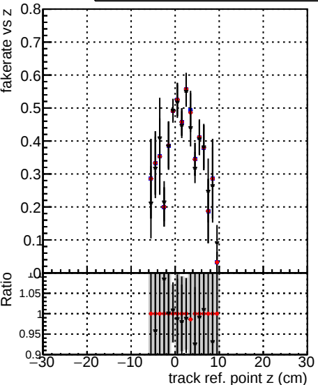
Fake rate vs verpos DOM TT original time DOM TT original time2 DOM TT modified time2
