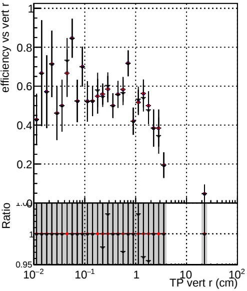
Efficiency vs vertpos DQM_TT_original_time DQM_TT_original_time2 DQM_TT_modified_time2
