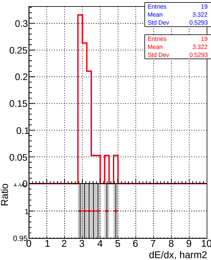
dE/dx estimator 1
