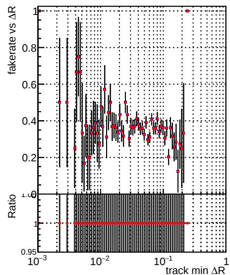
—•— DQM_TT_original_time —•— DQM_TT_modified_time
