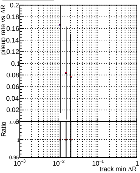
Legend: \bullet DQM TT original_time \bullet DQM TT newscoreonlyINIT_time \bullet DQM TT modified_time
