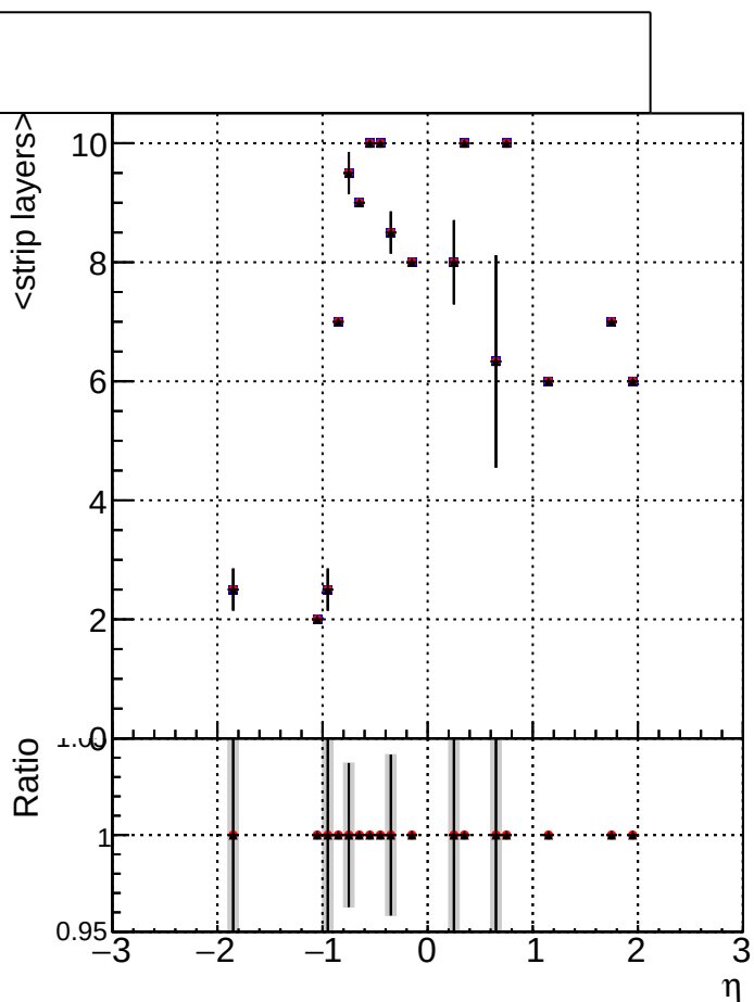
mean # STRIP hits vs eta
