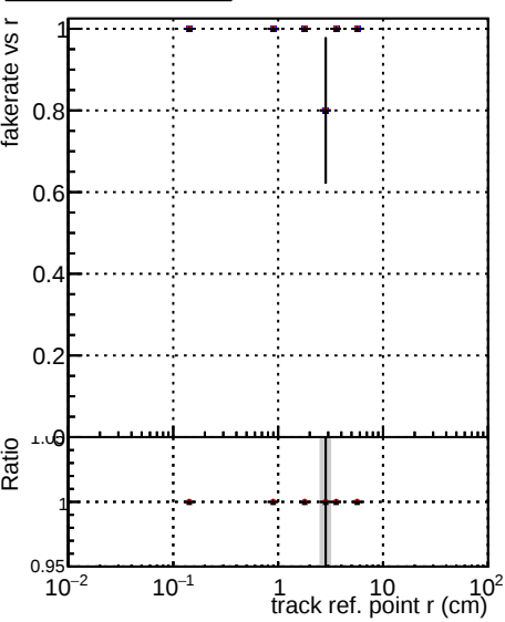
Fake rate vs verpos Legend: DQM TT original_time DQM TT newscoreonlyINIT_time DQM TT modified_time
