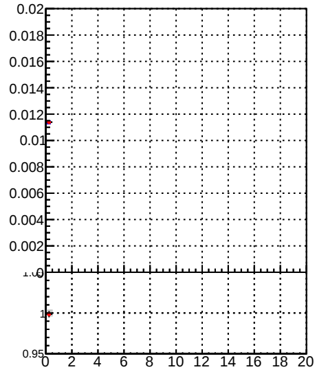
Fake rate vs. — DQM TT mkFit-DQM_original — DQM TT mkFit-DQM_modified5
